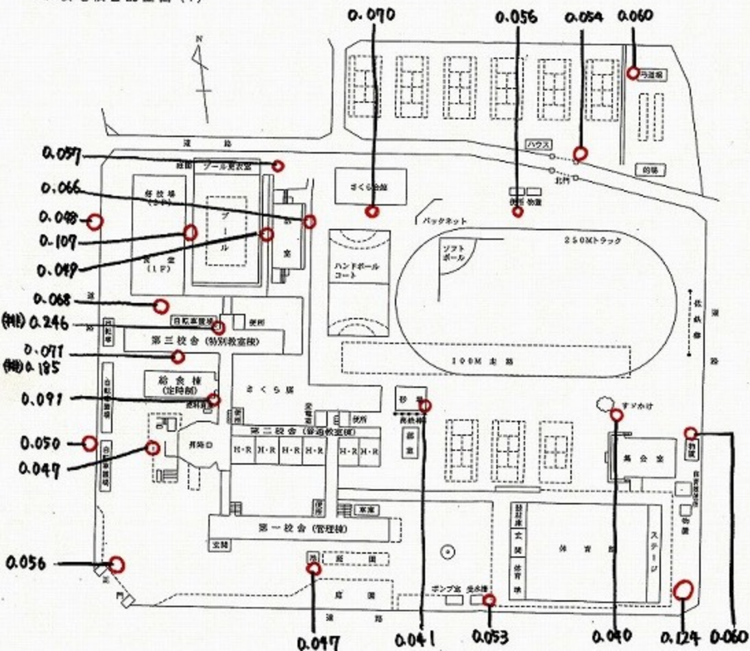
14. 校地校舎配置図(1)
